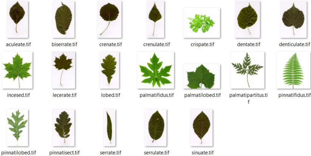
Fig. 2. Dataset
